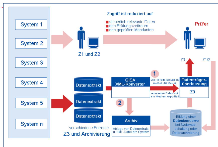
Lösungskonzept Z3-Zugriff: Datenextraktion
